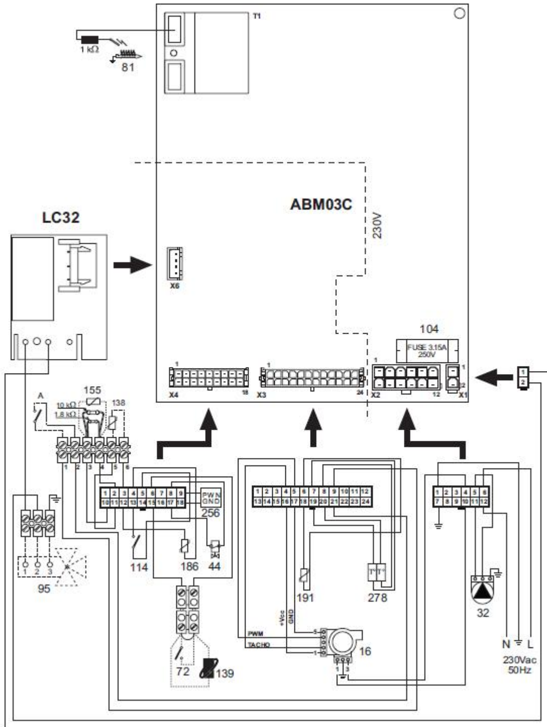
29. ábra - Elektromos kapcsolás
