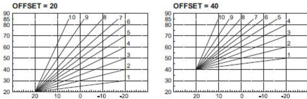
11.ábra - Különböző meredekségű követési görbék és párhuzamos eltoláson
