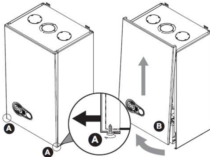
24. ábra - Elülső burkolat levétele
