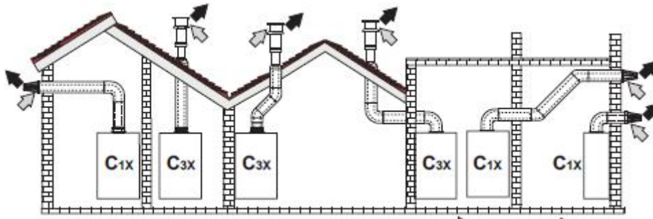
15. ábra - példák koncentrikus vezetésekre (→ =levegő, → =füstgáz)
